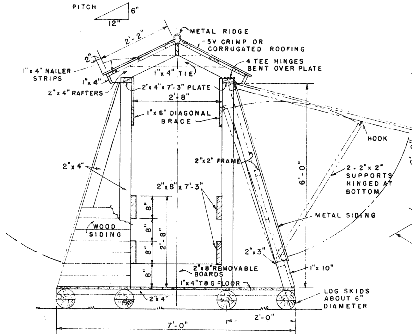
END ELEVATION
