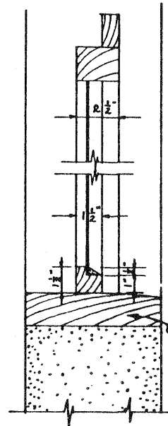
SECTION A-A
