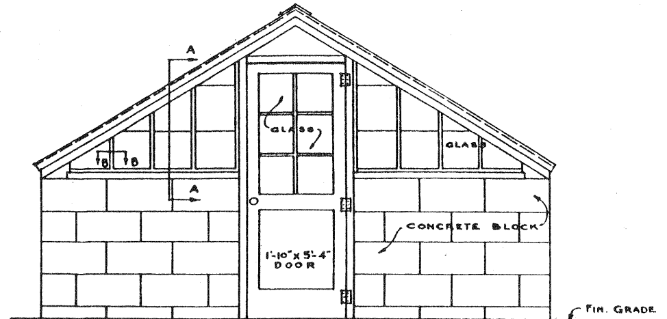
END ELEVATION
